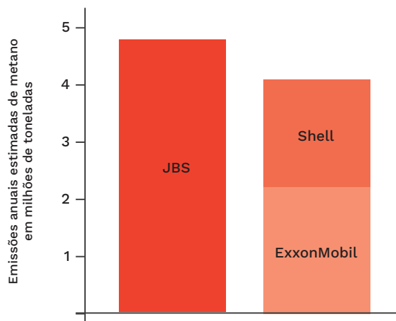
Gráfico 1: estimativa de emissões de metano da JBS comparado à combinação das emissões da ExxonMobil e Shell. Fonte: Greenpeace Nórdico (2024)
